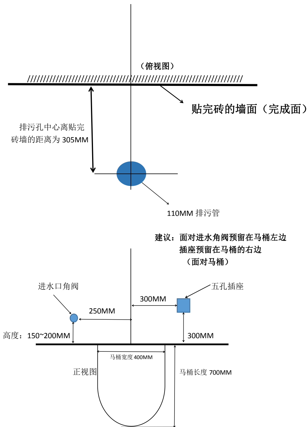
智能马桶安装预留水、电、坑距示意图
