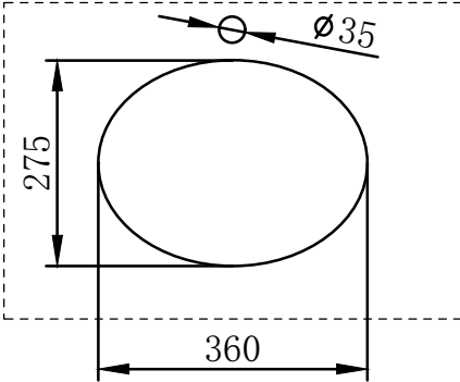
石板开孔尺寸图
