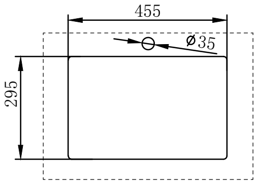
石板开孔尺寸图
