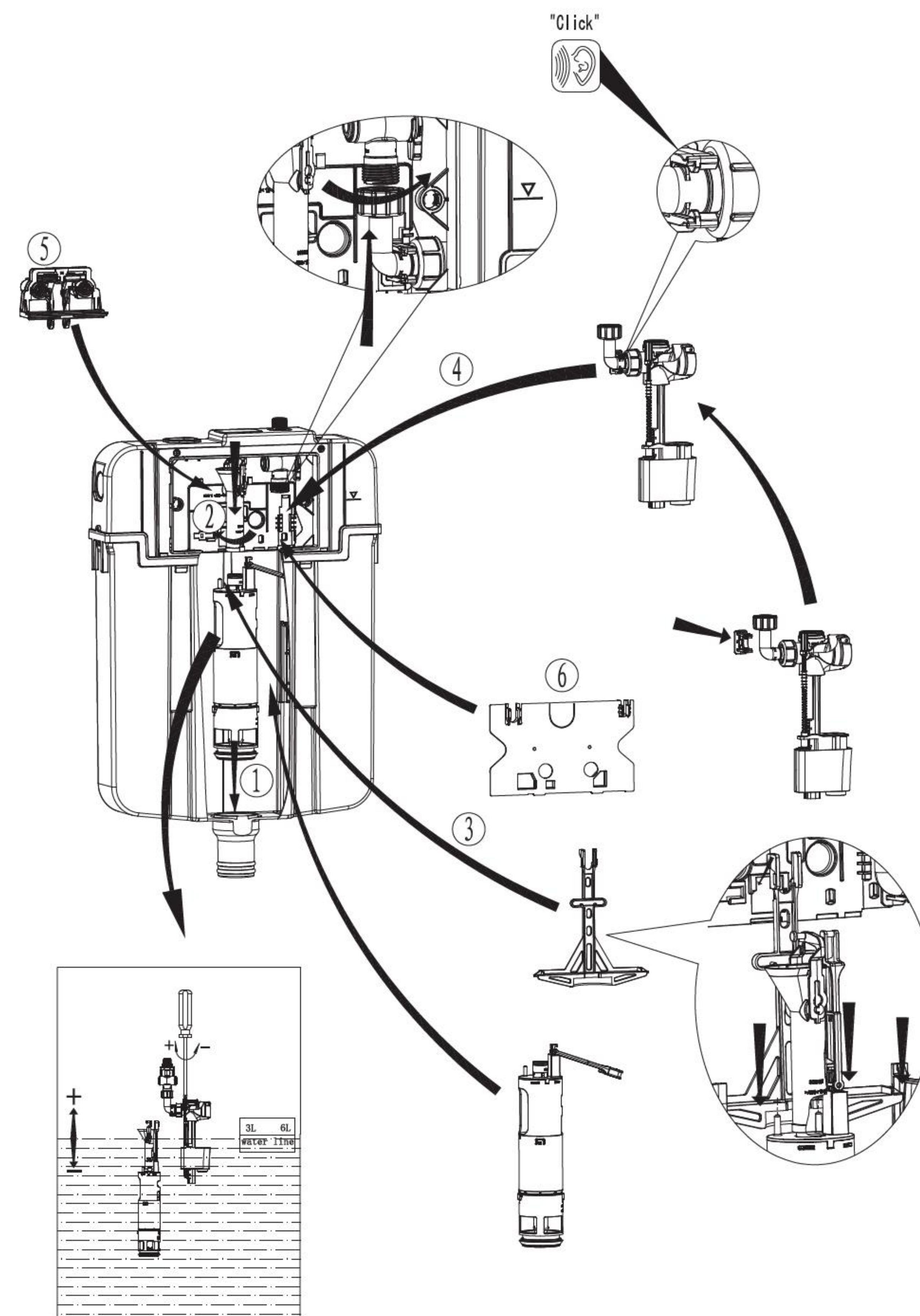
七、水箱配件安装图:
