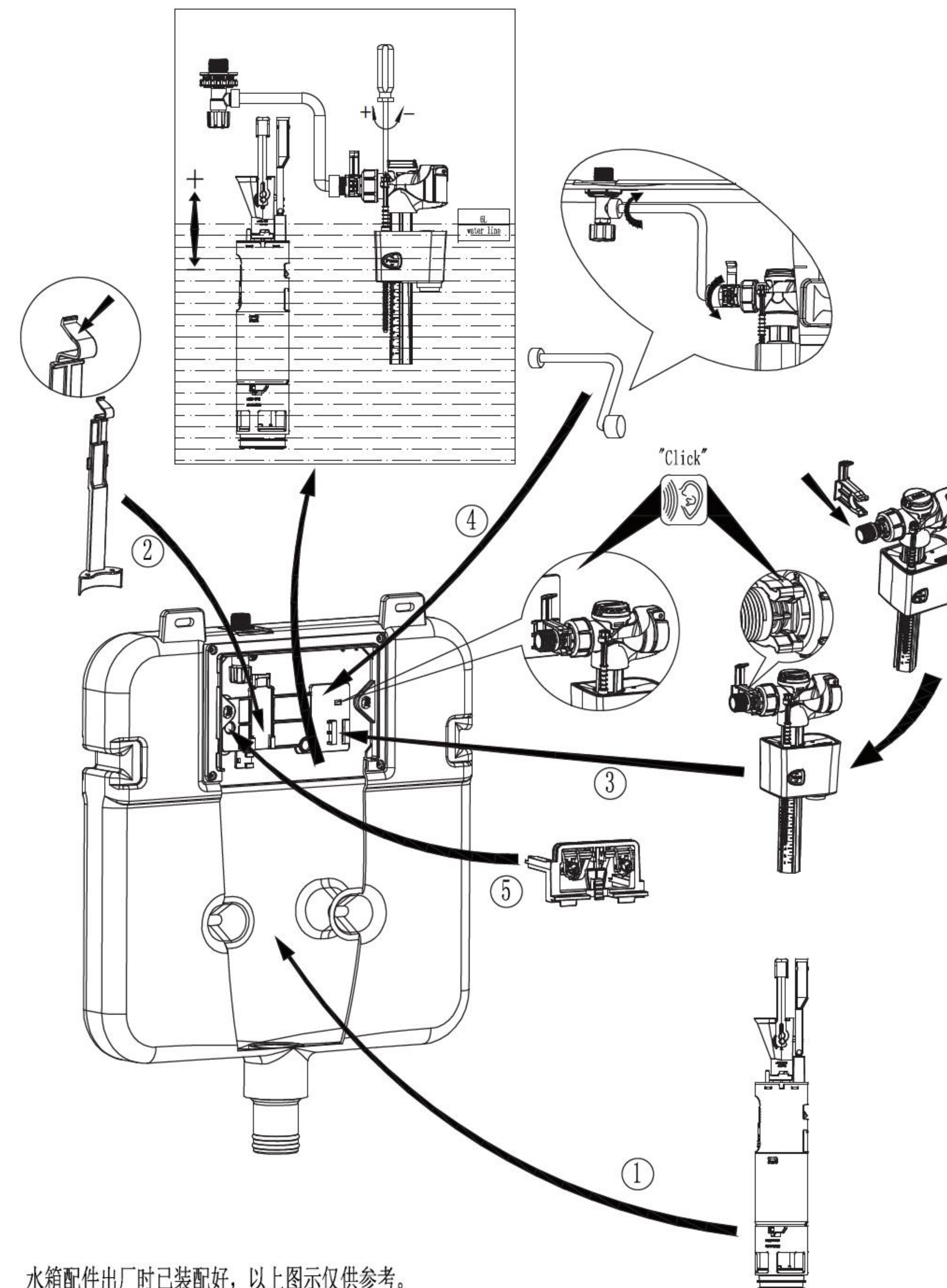
八、水箱配件安装图:
